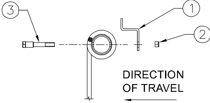
DETAIL A-A
